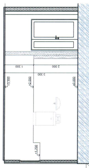
Rez A-A - pôvodný stav
